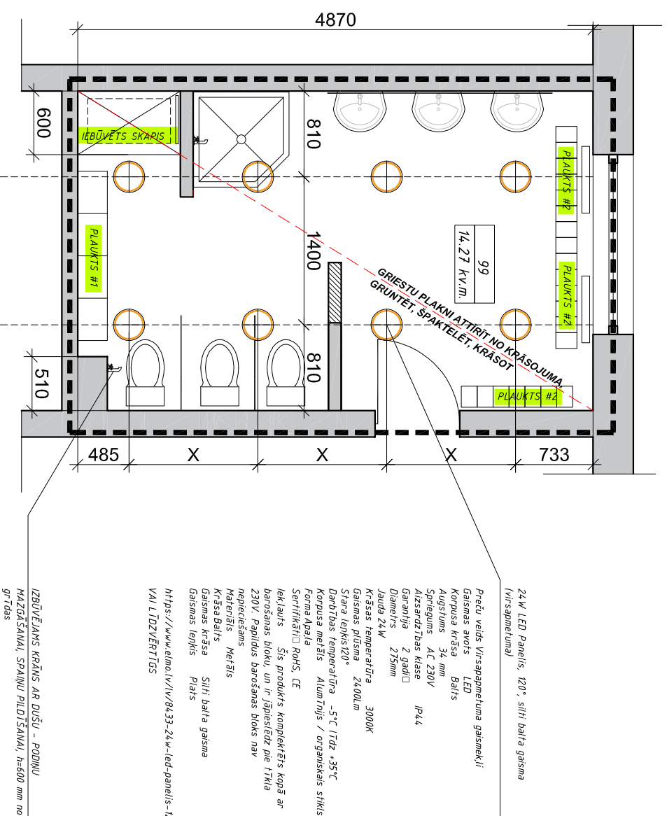
GRIESTU PLĀNS M1:50
