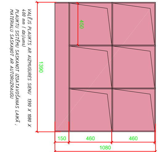
PLAUKTIS #1 M1:25
