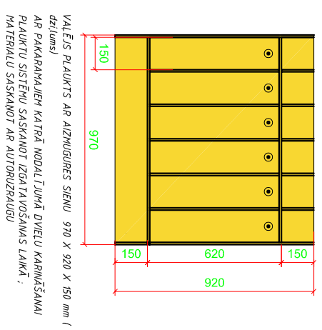
PLĀUKTS #2 M1:25
