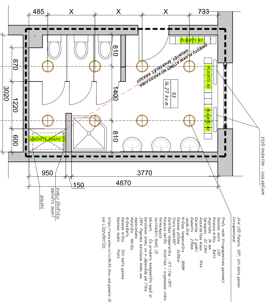
TELPAS Nr. 93 PĀRPLĀNOJUMS, PIEŠAISTES
