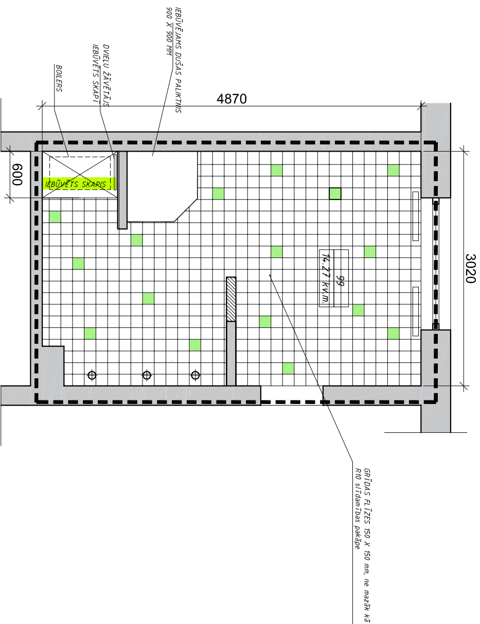
GRĪDAS PLĀNS M1:50
