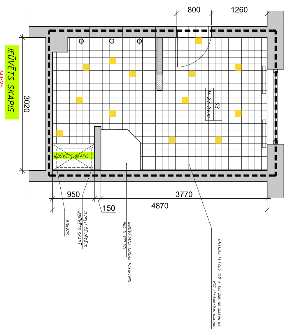
GRĪDAS PLĀNS M1:50
